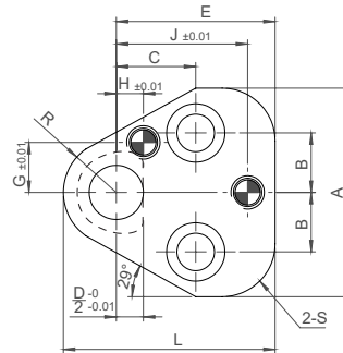
สำหรับพันชักรูปร่าง for Shaped Punch Model: 25DRFN25
