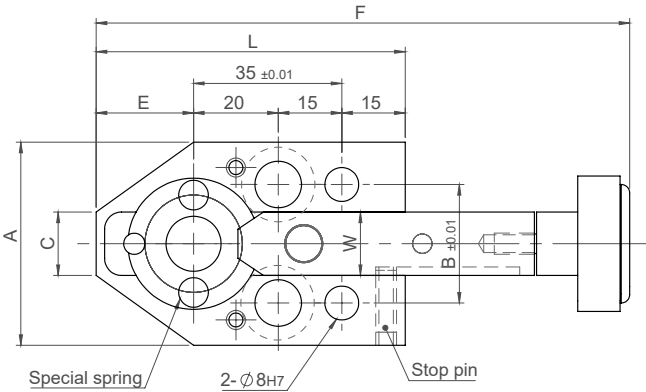
สำหรับพันซ์รูปร่าง for Shaped Punch Model: 25SLA-FH
