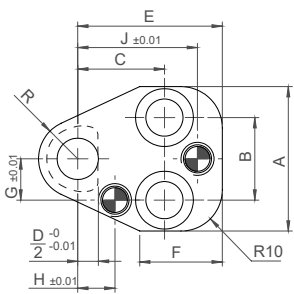
สำหรับพินรูปร่าง for Shaped Punch Model: 25ERFN
