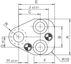
สำหรับพินกลม for Round Punch Model: 25ERAN
