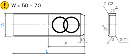
แบบไม่มีรูสกรู Without bolt holes Model: 25SGO
