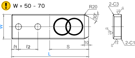
แบบมีรูสกรู With bolt holes Model: 25SGOA / 25SGOB
