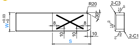
แบบไม่มีรูสกรู Without bolt holes Model: 25SGW
