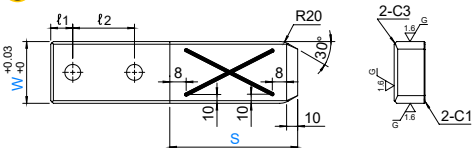
แบบมีรูสกรู With bolt holes Model: 25SGWA / 25SGWB
