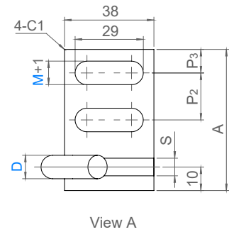
Model: 25SRG-R เสาด้านขวา Right Hand Type
