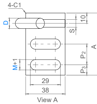
Model: 25SRG-L เสาด้านซ้าย Left Hand Type
