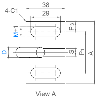
Model: 25SRG เสาด้านกลาง Center Type
