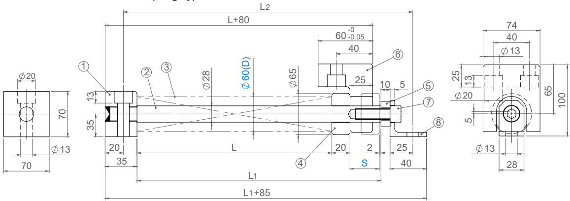
รุ่นสปริงชิ้นเดียว One Spring Type
