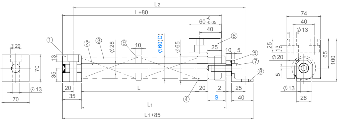
รุ่นสปริงสองชิ้น Two Spring Type
